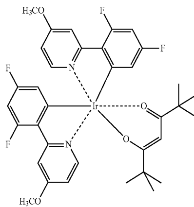
(F_2ppy)_2Ir(tmd)
