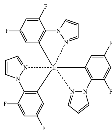
Ir(dfpz)_3
